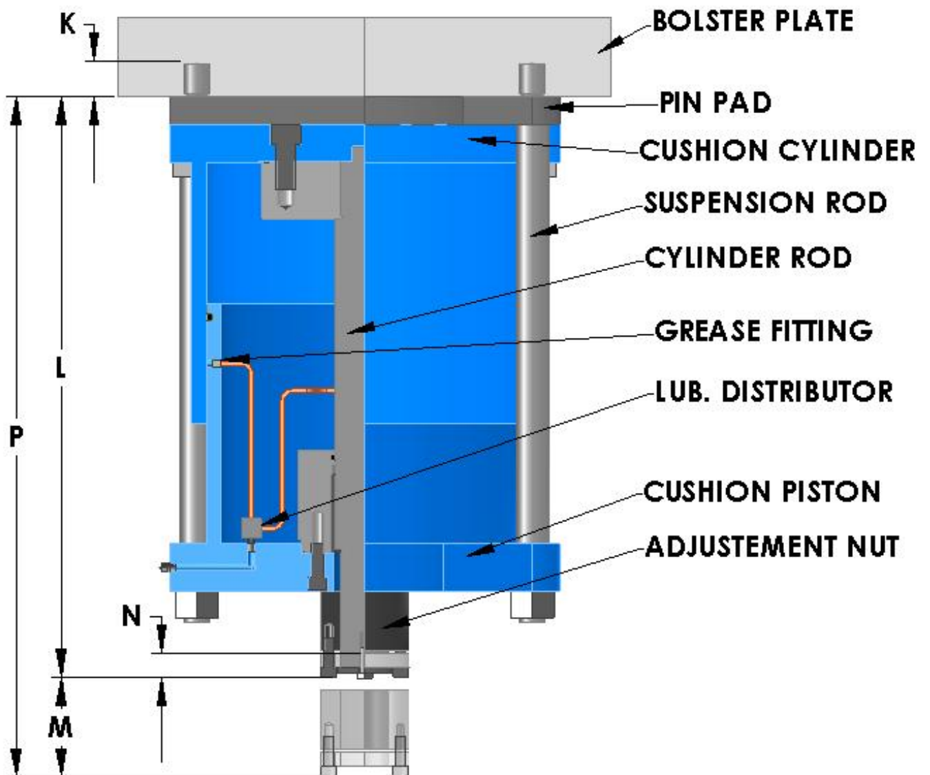
Fig. 4 BPM Model HD Die Cushion
